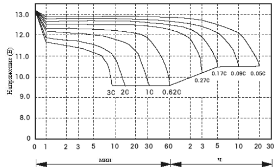
РАЗРЯДНЫЕ ХАРАКТЕРИСТИКИ (25°C)
